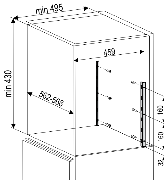
Montážna schéma dvojpolicový
